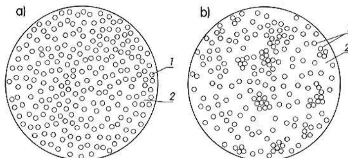
Rys. 6. Mikroskopowy obraz farby: a) dobrze zdyspergowany pigment, b) źle zdyspergowany pigment, [6, s. 52]
