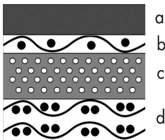
Rys. 9. Guma offsetowa kompresyjna [http://pl.wikipedia.org/wiki/Grafika:Blanket.svg] a – guma, b – tkanina stabilizująca, c – warstwa kompresyjna), d – gruba tkanina stabilizująca
