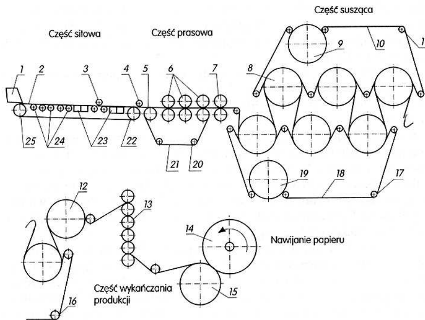
Rys. 1. Schemat maszyny papierniczej [11, s. 29]
