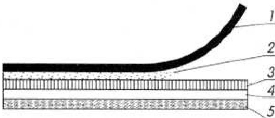
Rys. 8. Przekrój folii do tłoczenia [7, s. 184] 1 – nośnik, 2 – warstwa wosku (rozdzielająca), 3 – warstwa lakieru (ochronna), 4 – warstwa barwna, 5 – warstwa kleju (adhezyjna)
