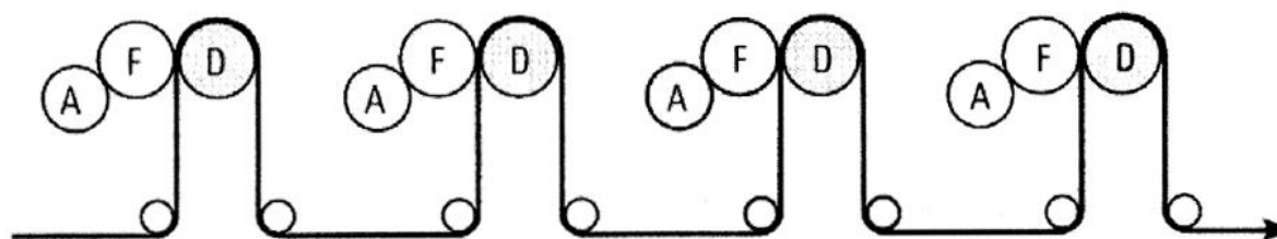
Maszyna fleksograficzna 4-kolorowa, zwojowa
