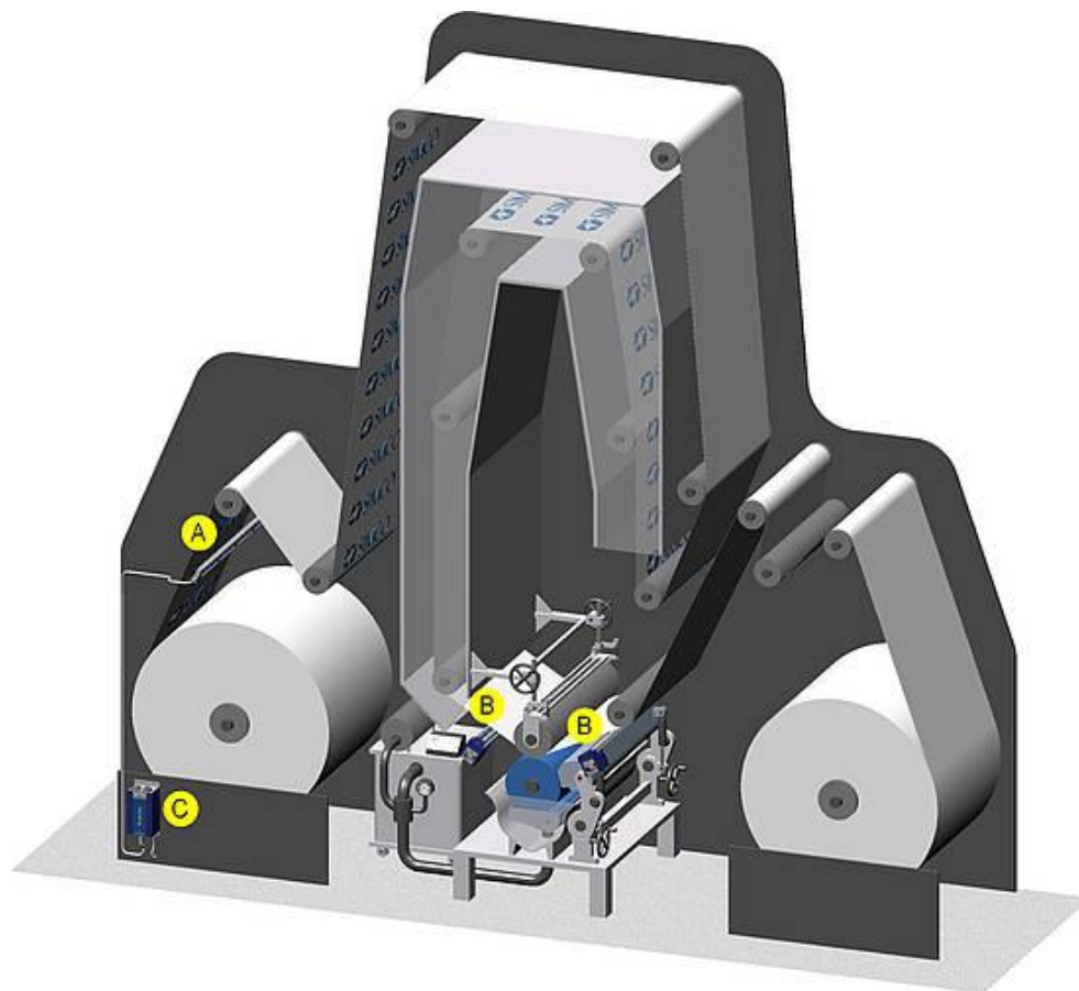
maszyna rotograviurowa
